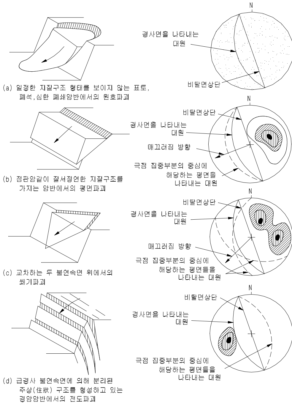
[그림 11.6] 암반사면의 파괴 유형별 평사투영해석 예시
