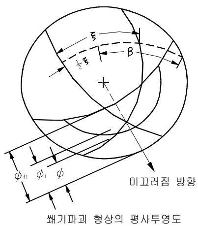
[그림 11.8] 빼기파괴 활동면 및 사잇각 산출 방법
